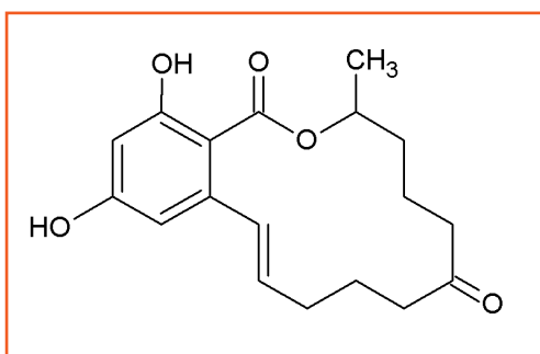
Kuva 3. Zearalenonin rakenne
