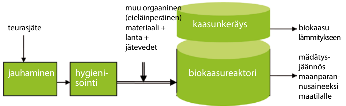
Kuva 7. Maatilan yhteydessä oleva biokaasulaitos
